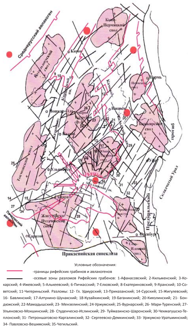
Рис. 1. Тектоническая схема Волго-Камской антеклизы
